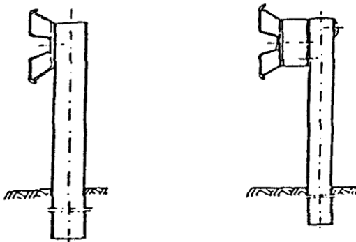
Załącznik 11.3. Zasady określania wysokości prowadnicy bariery nad poziomem terenu, wg [32]
