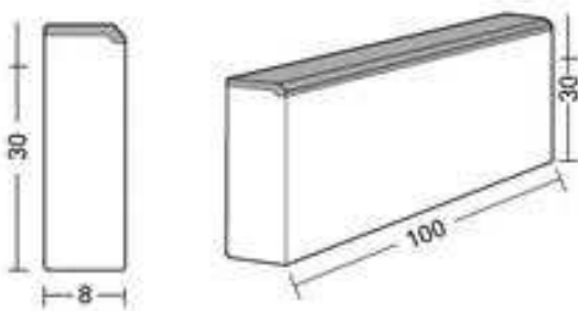
Rysunek 1. Kształt betonowego obrzeża chodnikowego
